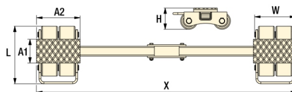
Pattino doppio con binario serie EMLSD
